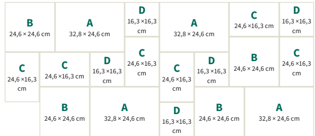
Wilder Verband 3
