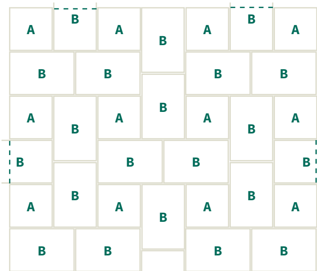
Kreuzverband
